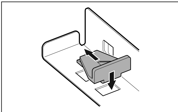
Fig. 61 Τοποθέτηση γωνίας τερματισμού
