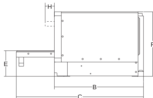
Forni sovrapponibili Stackable ovens
